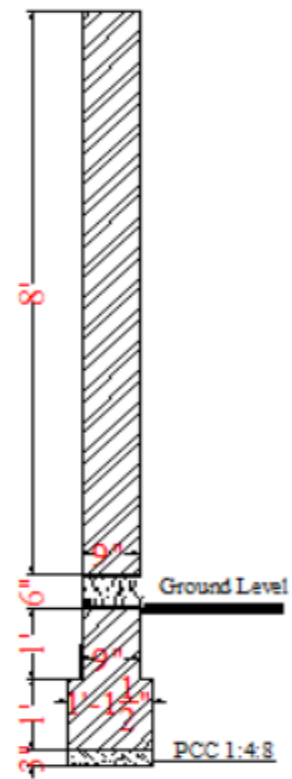
Toilet Wall Section
