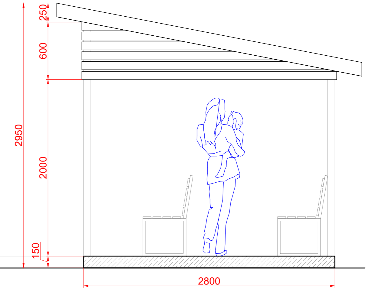
Вид збоку
